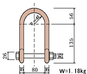
テトラシャックル φ16mm
