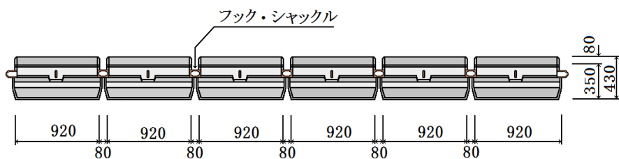
テトラシャックル φ16mm
