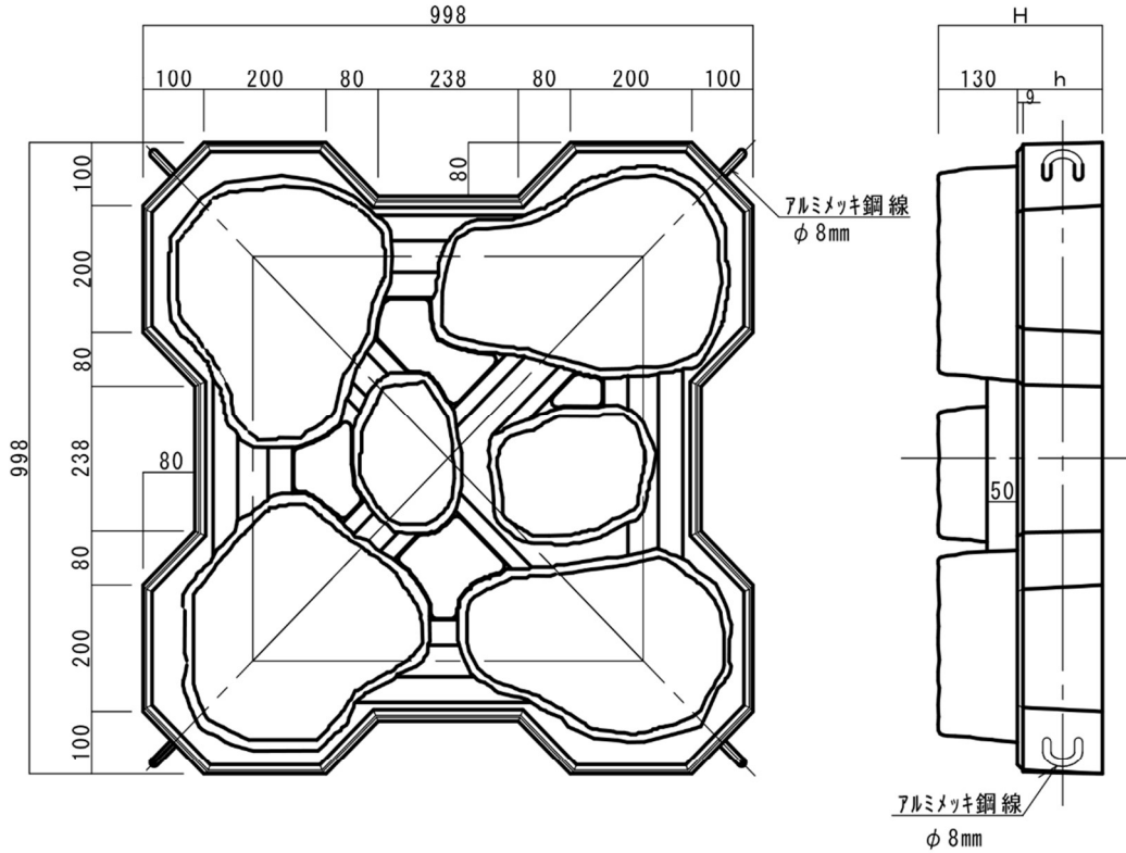
連結部詳細
