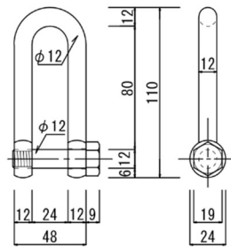
ネジシャックル寸法図
